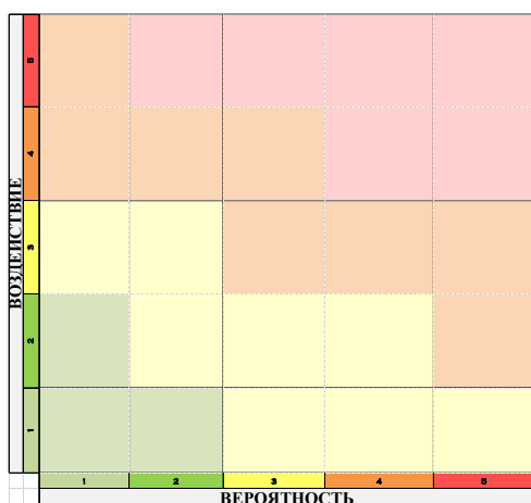
Рисунок 3 – Карта рисков
